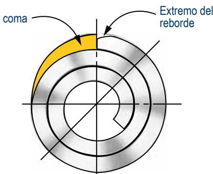
El extremo del reborde está diseñado para esconderse dentro del diámetro del orificio.
