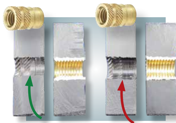
Figura 1 Flujo de plástico correcto
